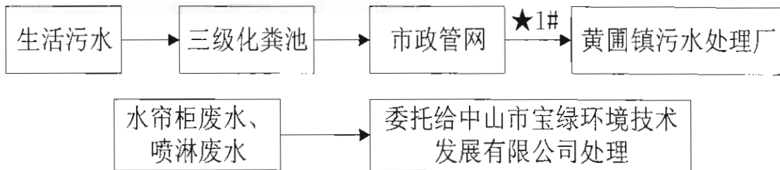
图3-1 废水处理工艺流程图
