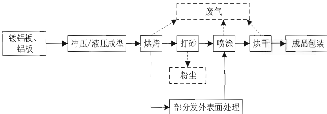
图 2-2 电饭锅内胆、小烤箱（外壳）生产工艺流程图
