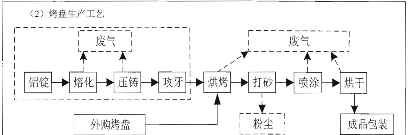
图 2-3 烤盘生产工艺流程图
